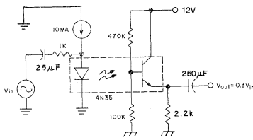
Fig. 99 - Linear A.C. coupler.
