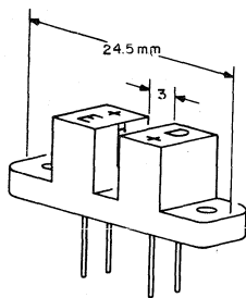
Fig. 10a - Interrupter module.
